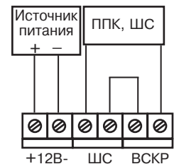
Рисунок 3 – Схема подключения извещателя с объединенными шлейфами сигнализации и вскрытия корпуса
